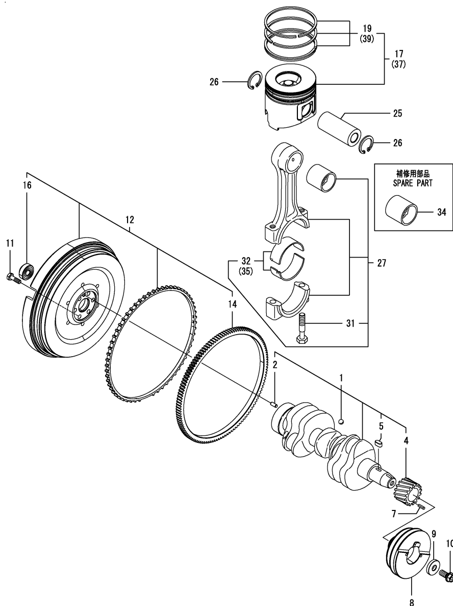
Fig.10. CRANKSHAFT & PISTON
