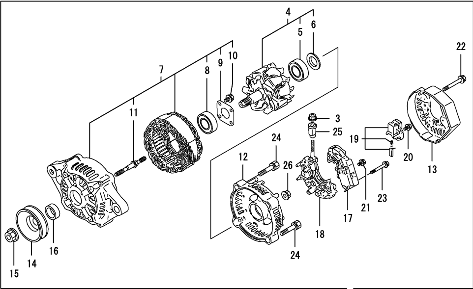
Fig.18. GENERATOR
