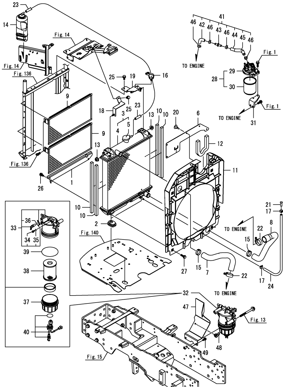
Fig.2. RADIATOR
