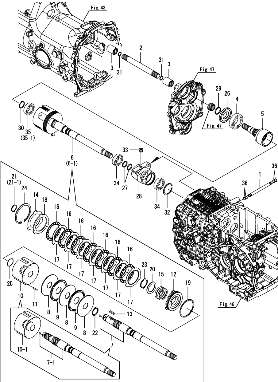
Fig.50. P.T.O. CLUTCH
