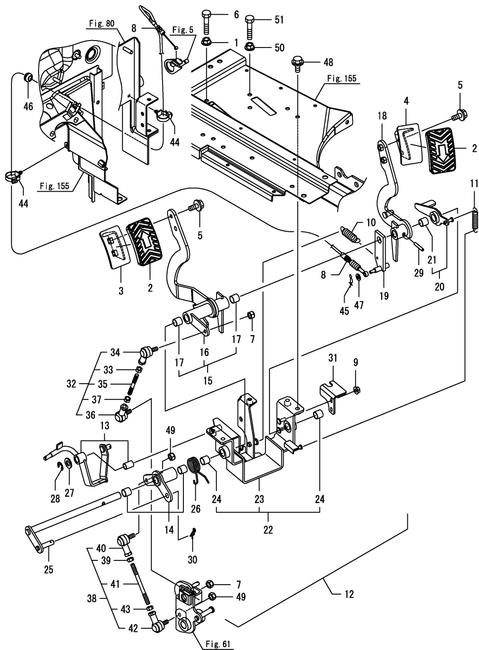
Fig.62. H.S.T. CONTROL
