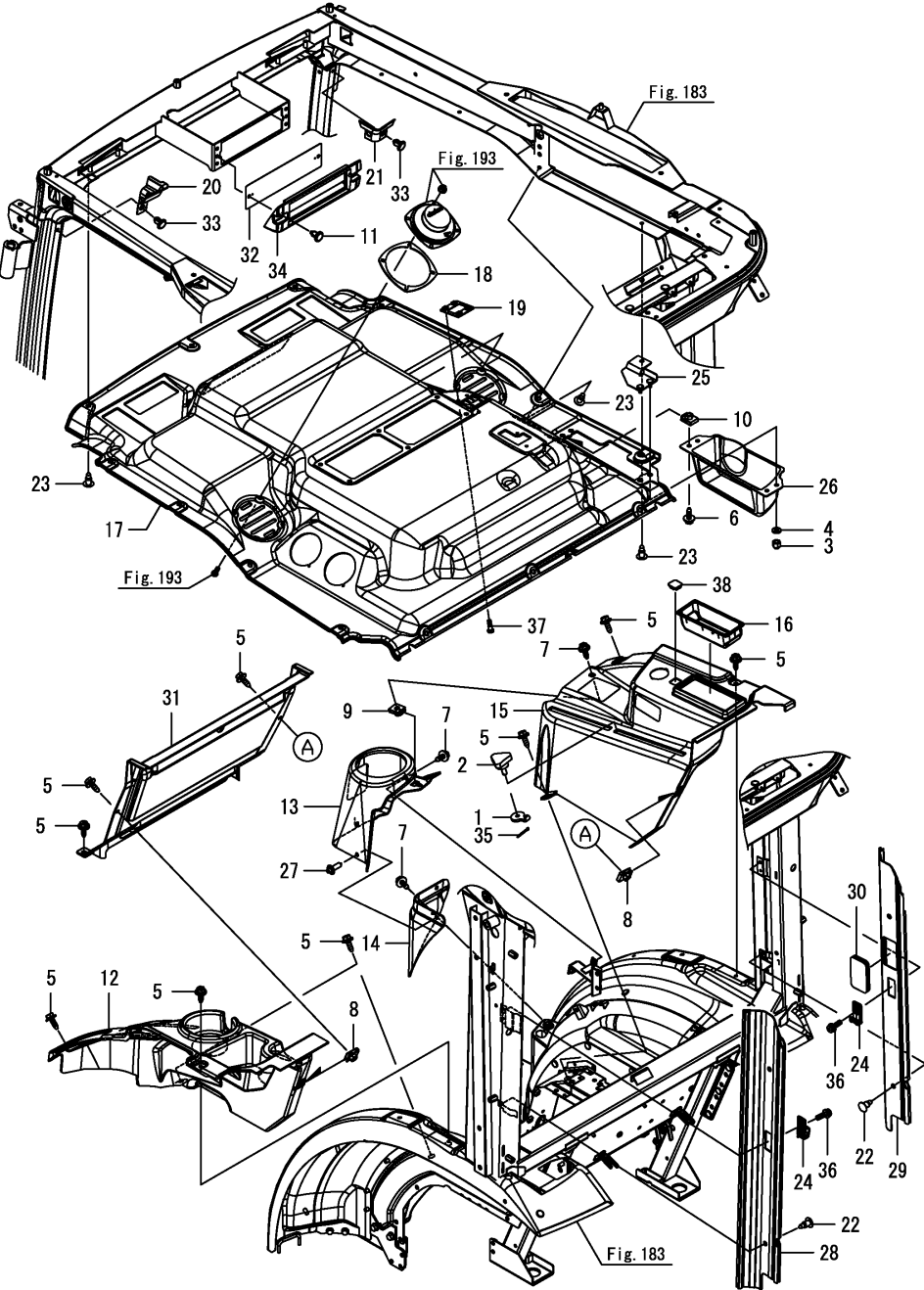
Fig.151. INTERIORS(CABIN)
