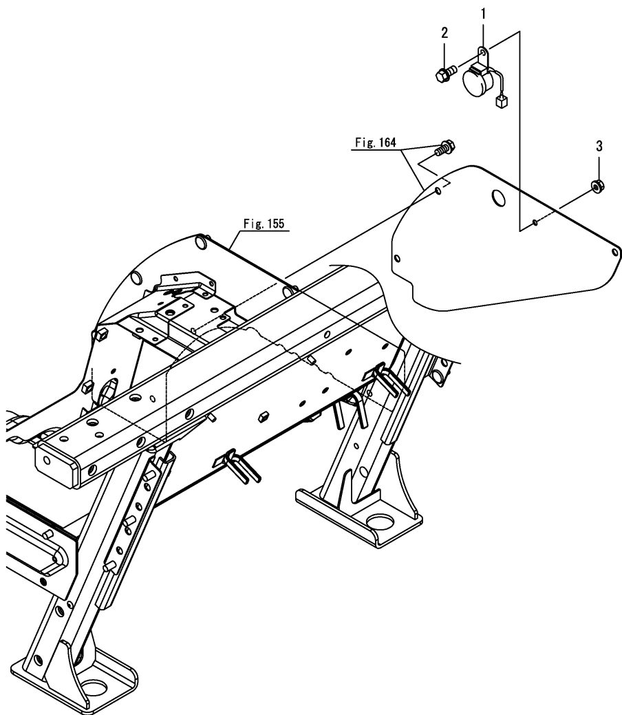
Fig.128. BACK BUZZER
