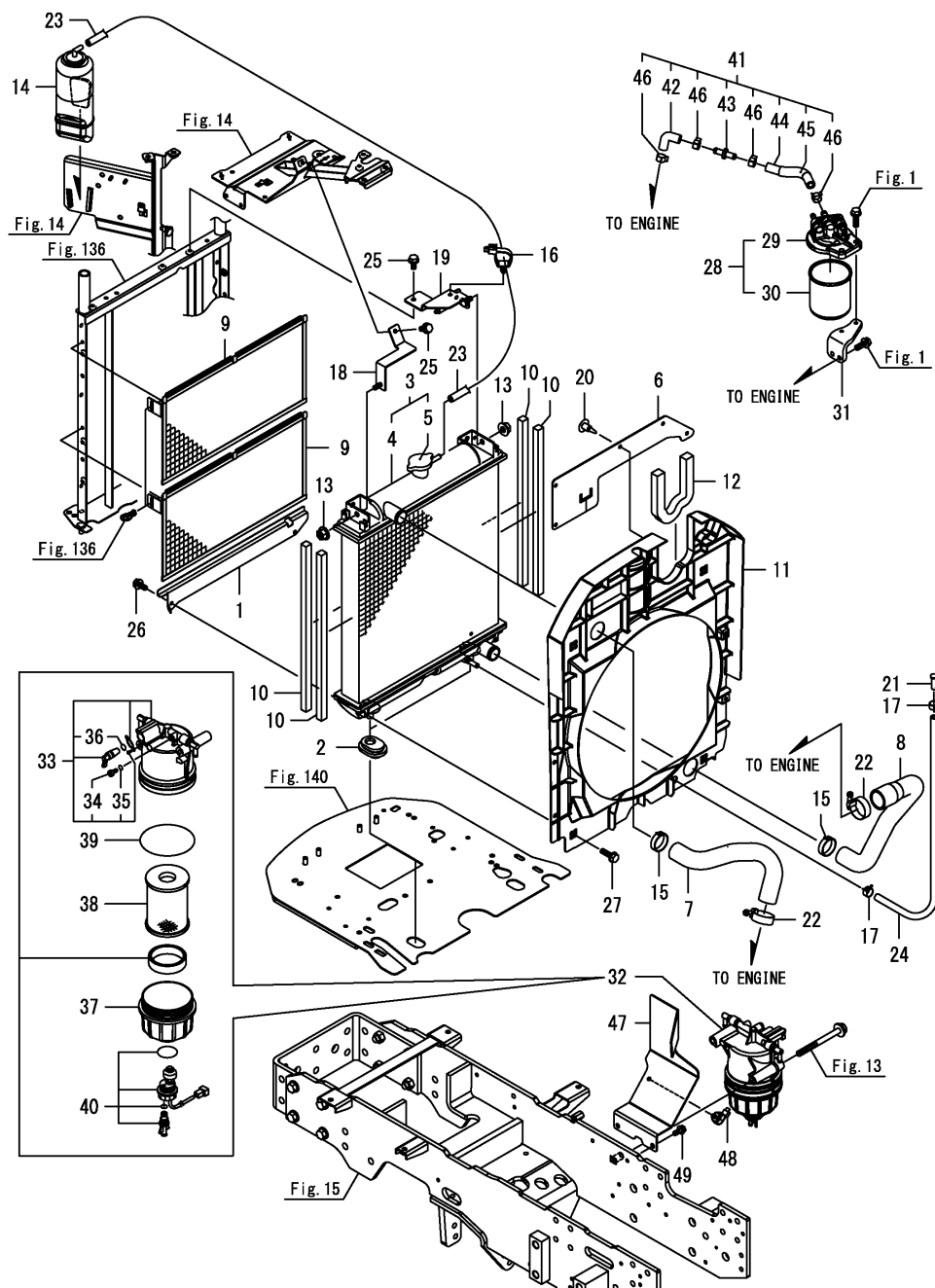
Fig.2. RADIATOR
