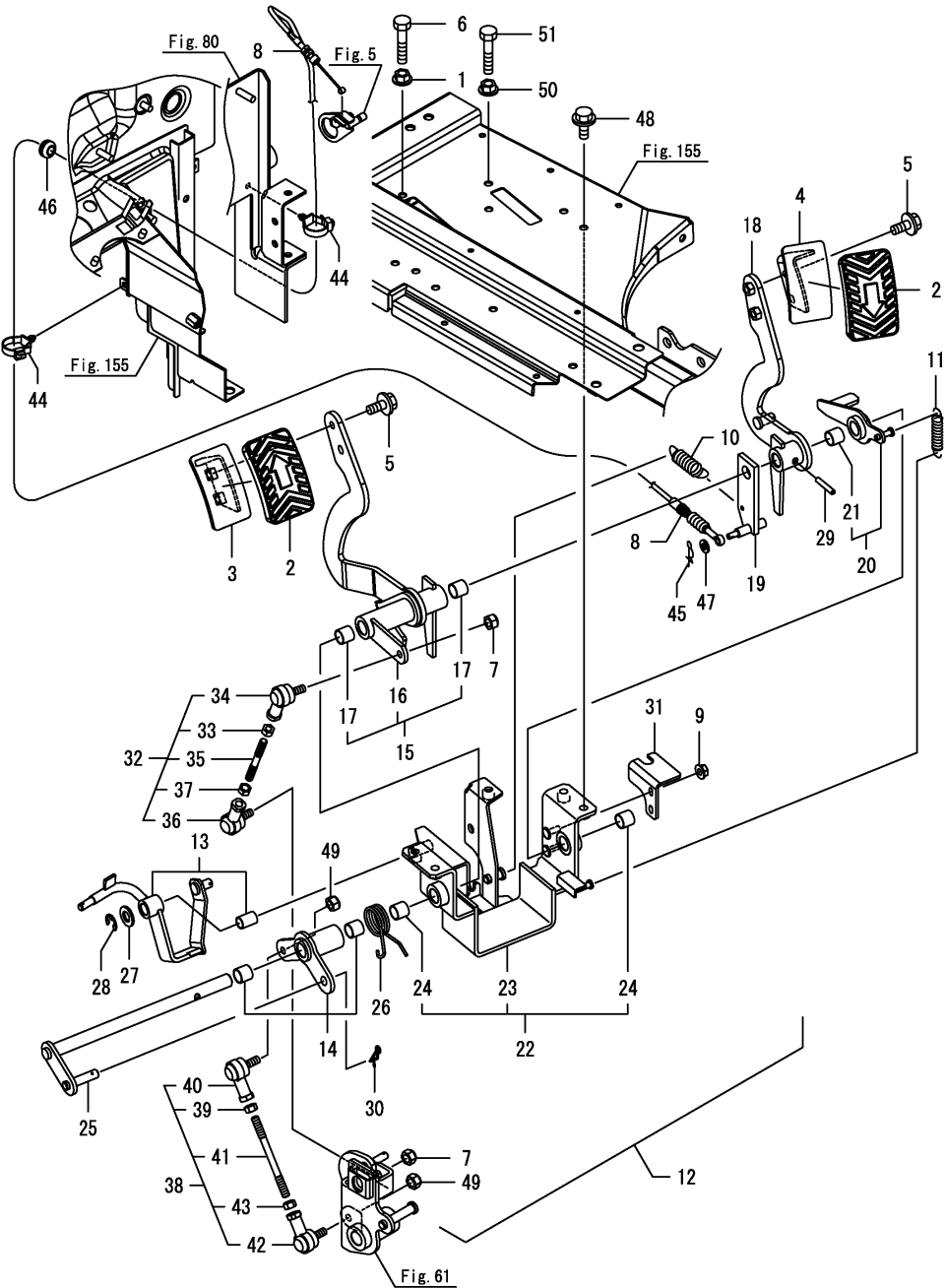
Fig.62. H.S.T. CONTROL
