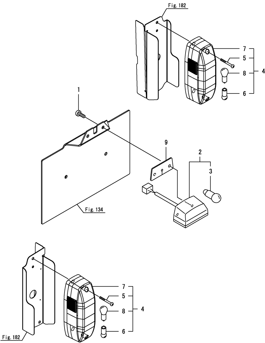
Fig.120. LAMP(FLOOR)(REAR)(CABIN)
