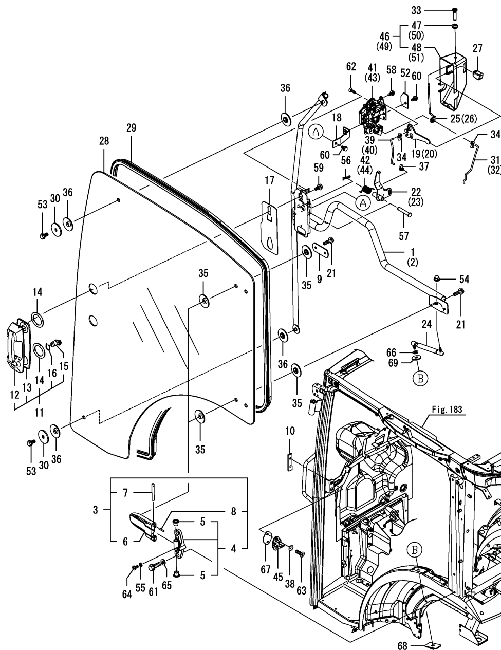
Fig.184. DOOR
