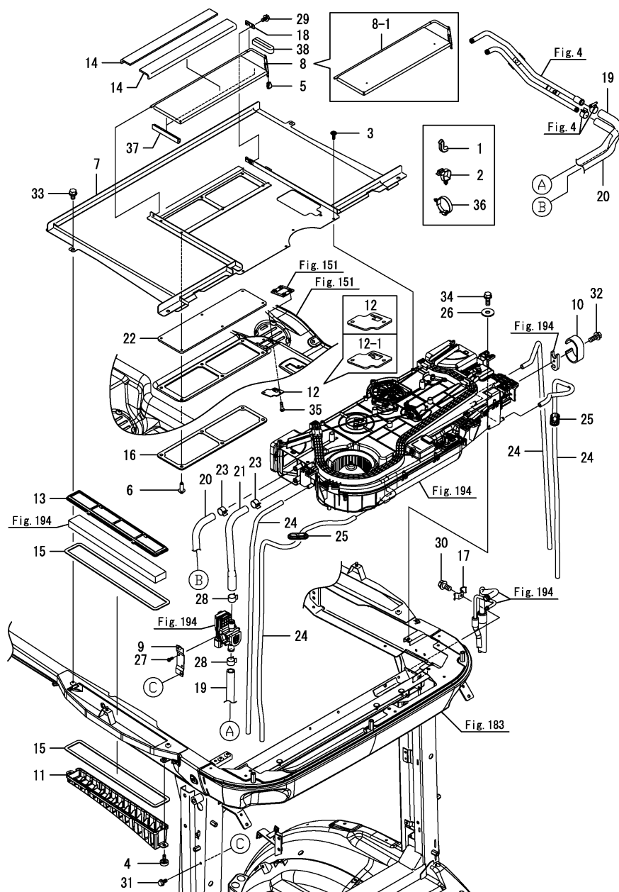
Fig.196. AIR CONDITIONER(3)
